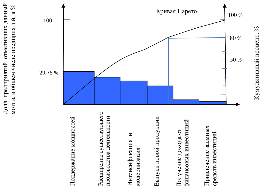
Рис. 2. Диаграмма Парето
