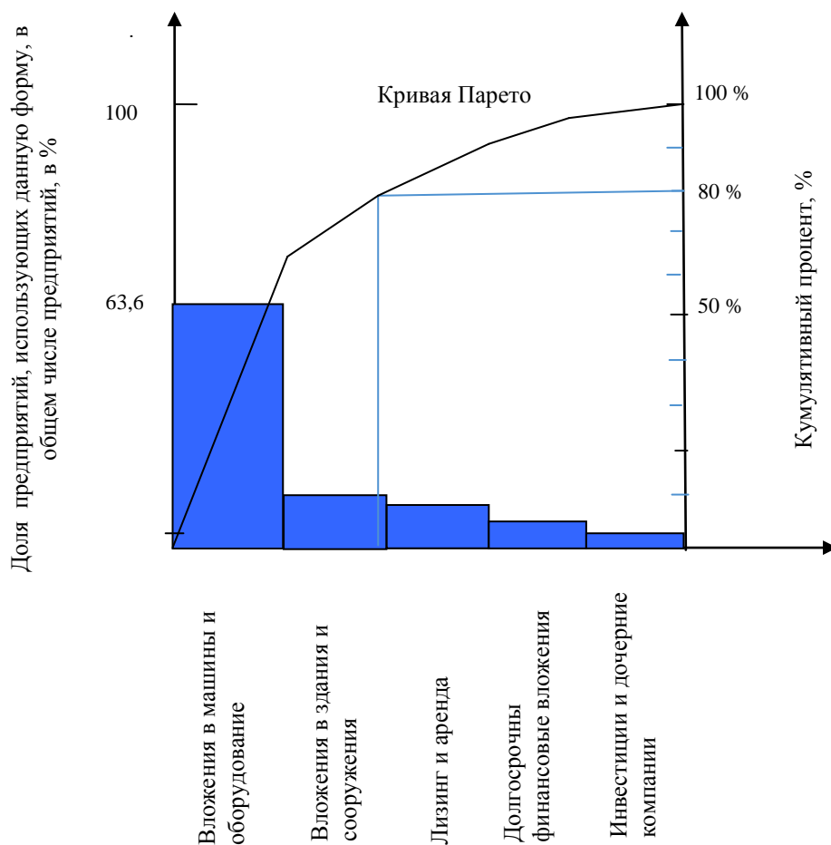
Рис. 3. Диаграмма Парето
