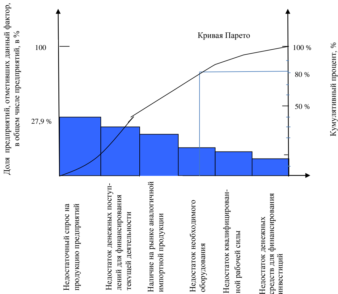
Рис. 1. Диаграмма Парето
