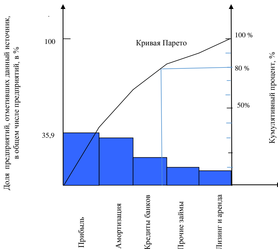
Рис. 4. Диаграмма Парето
