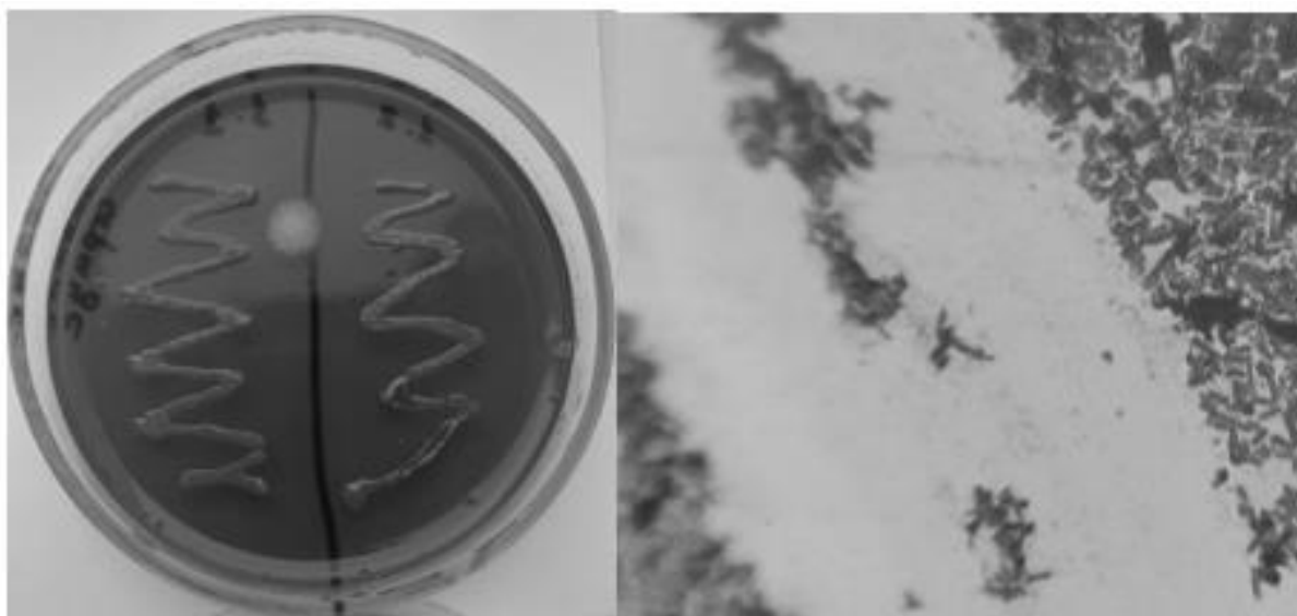
Рис. 3. А – выросшие колонии на среде Эндо, Б – обнаруженные грамположительные палочки ( \times 1200 )
