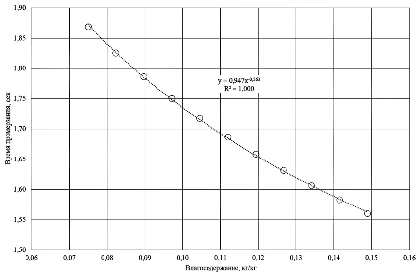
Рис. 5. Расчет времени, необходимого для криогенного замораживания семян кориандра
