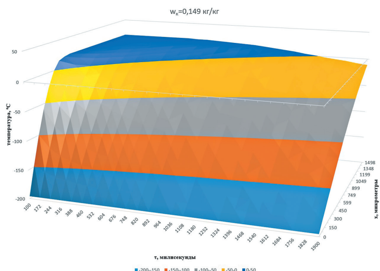
Рис. 4. Кинетика температурного поля криогенного замораживания семян кориандра при влагосодержании 0,149 кг/кг
