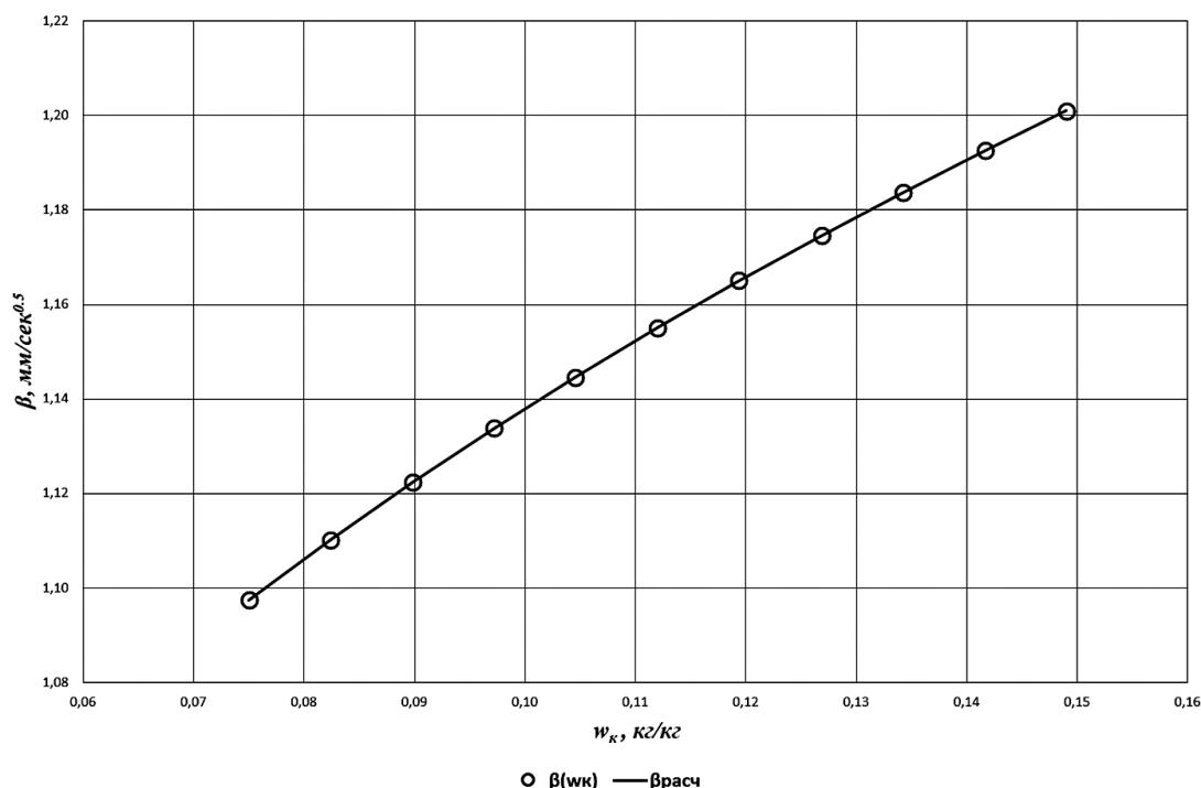
Рис. 2. Влияние влагосодержания на параметр характеристического уравнения процесса криогенного замораживания семян кориандра
