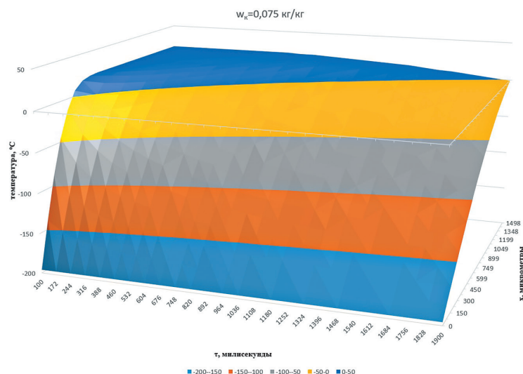
Рис. 3. Кинетика температурного поля криогенного замораживания семян кориандра при влагосодержании 0,075 кг/кг
